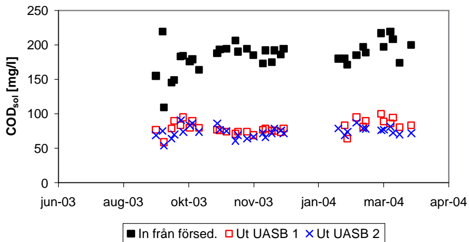
Figur 21. Lösligt COD (<math><0,45\mu\text{m}</math>) efter försedimenteringen samt ut från var och en av UASB-reaktorerna. Värderna för försedimenterat vatten är dygnsprover, prov från UASB-reaktorerna är stickprov.
