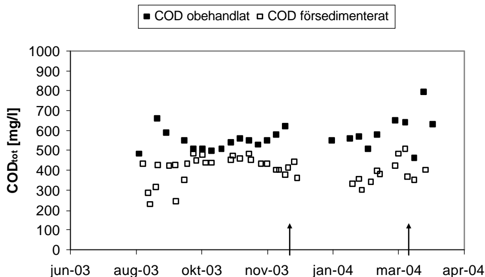
Figur 5. Totalt COD-innehåll i det obehandlade hushållsavloppsvattnet vid ankomsten till Sjöstadverket samt efter försedimentering. Pilarna visar tidpunkten för start av Purifixdosering 40 mg/l respektive 34 mg/l.
