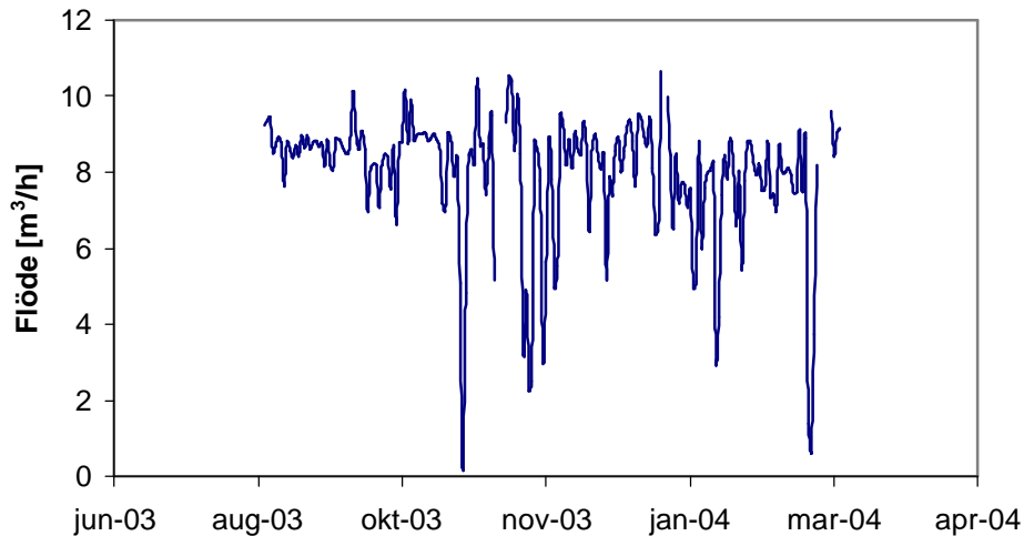
Figur 13. Dygnsmedelflöde till rens-galler Sjöstadverket.
