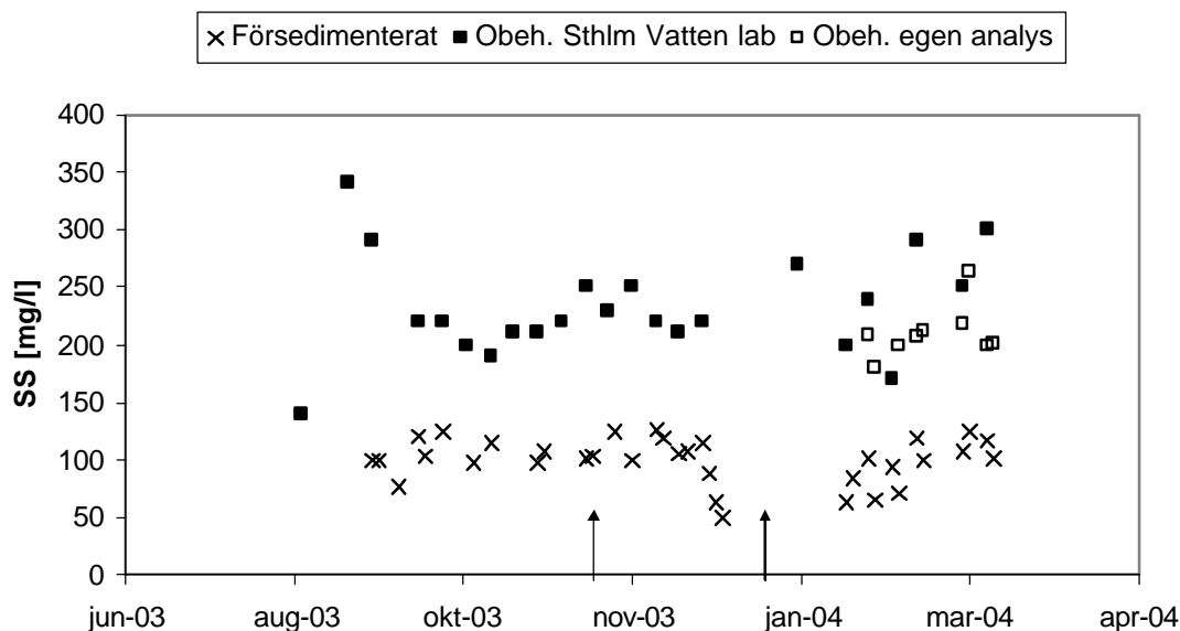
Figur 4. Total mängd suspenderat material ( >1,6\mu\text{m} ) i inkommande vatten till Sjöstadverket (värden från Stockholm Vattens lab. och egna analyser) samt i det försedimenterade vatten som motsvarar inflödet till UASB-reaktorerna. Pilarna indikerar start av Purifixdosering 40 mg/l resp. 34 mg/l.
