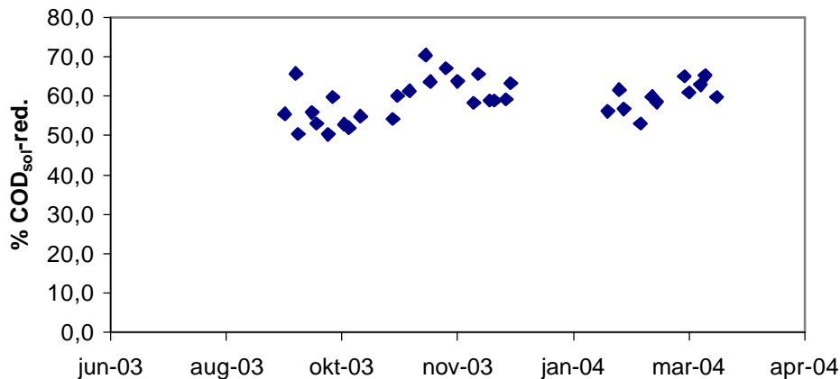
Figur 22. Reduktion av lösligt COD ( <0,45\mu\text{m}</math>) över UASB-reaktorerna.
