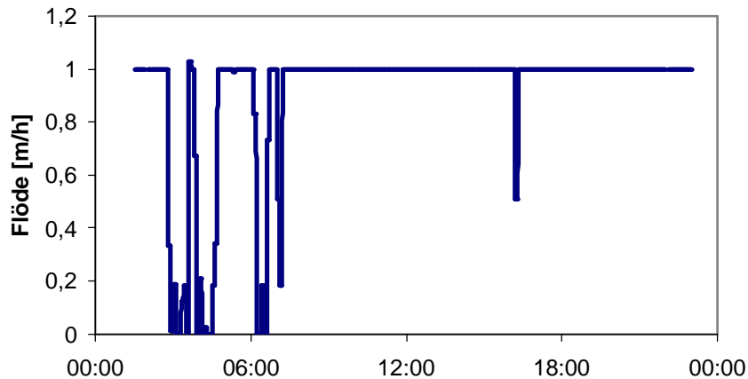
Figur 14b. Flöde in till försedimentering under ett dygn.
