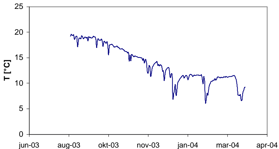
Figur 11. Temperatur i försedimenteringen på Henriksdalsverket (dygnsmedelvärden).
