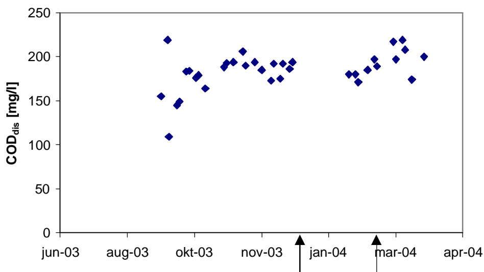
Figur 6. COD i inkommande vatten till UASB. Lösligt COD (<0,45 μm). Pilarna visar tidpunkten för start av Purifixdosering 40 mg/l den 18/12 2003 samt sänkning av dosen till 34 mg/l den 16/2 2004.
