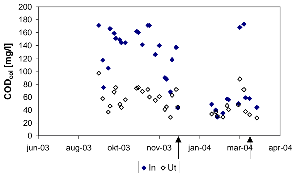
Figur 23. Kolloidalt COD efter försedimentering (dygnsprov) och efter UASB-reaktor två (stickprov från klarfasen). Pilarna visar tidpunkterna för start av Purifixdosering 40 mg/l respektive 34 mg/l.
