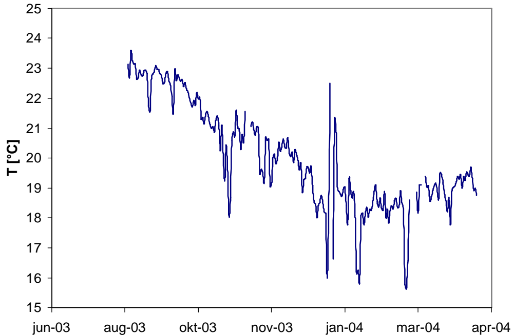
Figur 10. Temperatur i försedimenteringen före anaerob behandling (dygnsmedelvärden).
