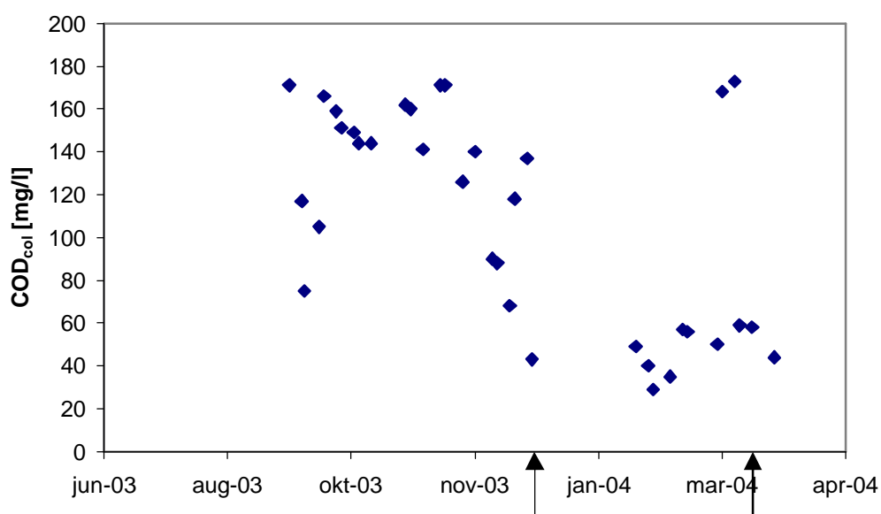
Figur 7. Kolloidalt COD (0,45 - 4,4 μm) i inkommande vatten till UASB. Pilarna visar start av Purifixdosering 40 mg/l respektive 34 mg/l.
