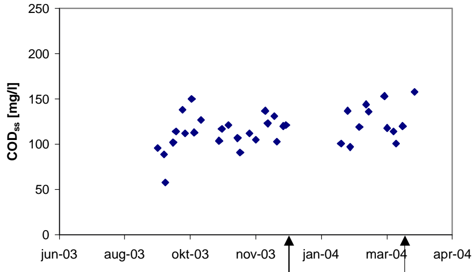
Figur 8. Suspenderat COD (>4,4 \mu m) i inkommande vatten till UASB. Pilarna visar tidpunkterna för start av dosering Purifix 40 mg/l respektive 34 mg/l.
